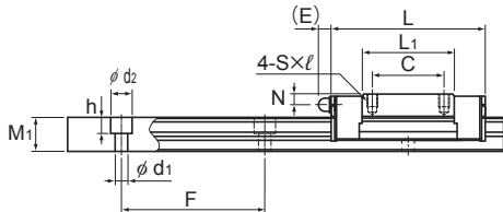
SRS15WGM/WGN型
