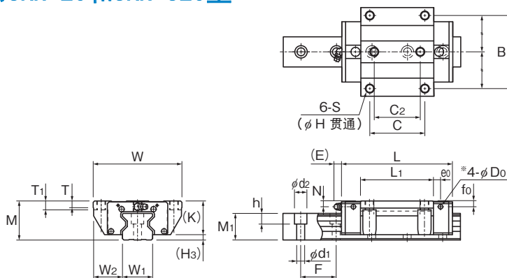
SRN35~65C/LC型
