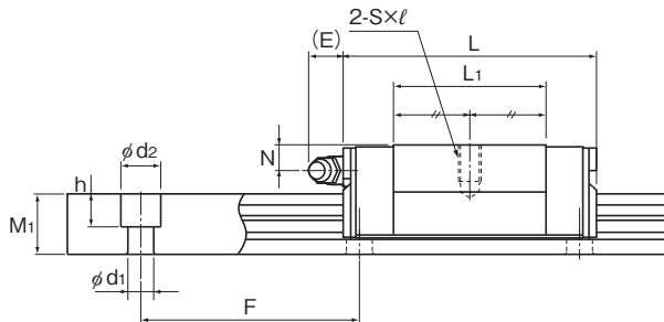
GSR15~25V型
