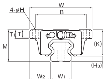
HSR20M1B/M1LB型
