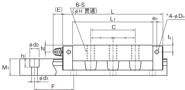
NR-LCX型
