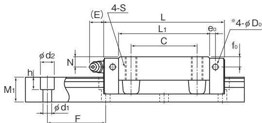
NR-A型、NRS-A型
