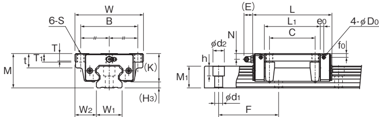
HSR45~85CA/HA/XCA/XHA型
