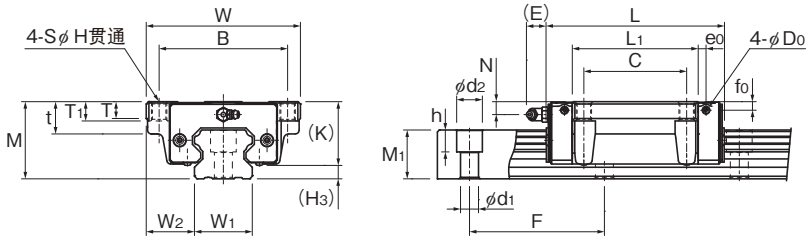
HSR45~65C/LC/XC/XLC型
