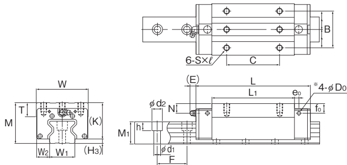
SRG35~65R/LR/LV型
