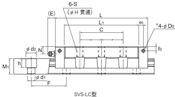
SVS-LC型
