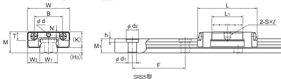
SRS5型
