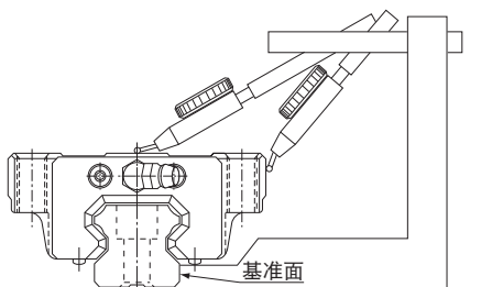
图15 行走平行度
