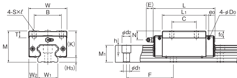
HSR45~85R/LR/XR/XLR型
