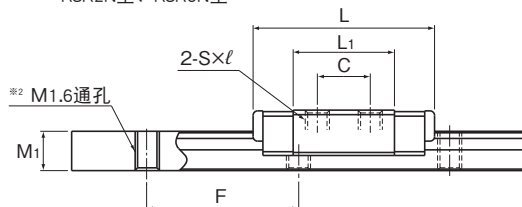
RSR3M型
