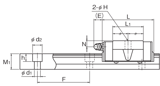
SR-M1SB型
