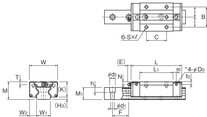
SRN35~65R/LR型
