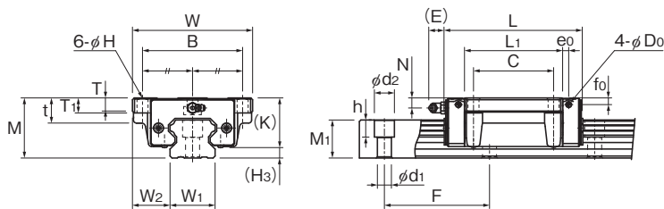
HSR45~85CB/HB/XCB/XHB型
