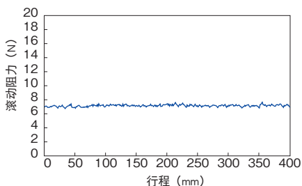
球保持器型LM滚动导轨 #25滚动阻力变动数据 (垂直使用、进给速度: 1mm/sec)
