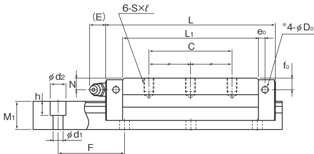
NR-LRX型
