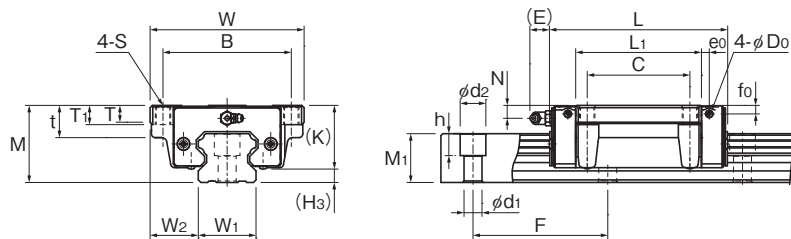
HSR45~85A/LA型
