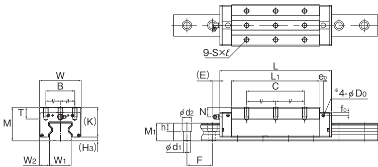
SRG35~55SLR型
