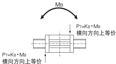
图4 M_b 力矩的等价系数
