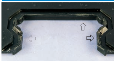
⇔ 标记箭头的区域为破裂之处
