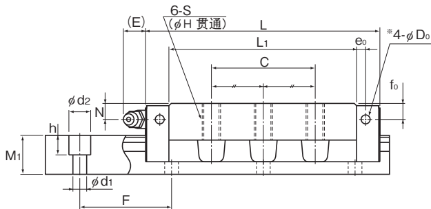
NR-LCX型
