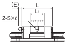
SRS15WGS型
