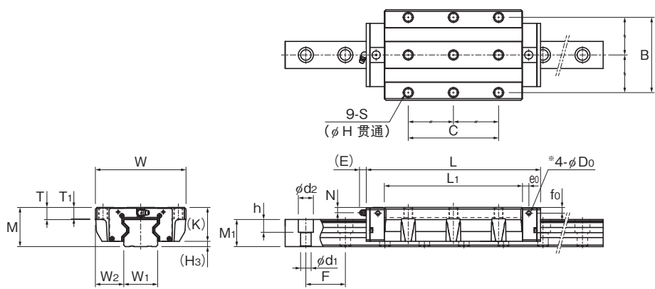
SRN35~65SLC型
