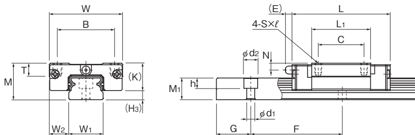
RSX15M型
