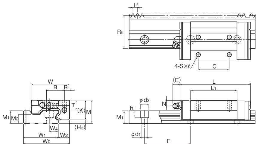
GSR-T-R型
