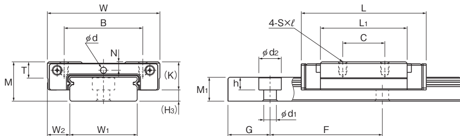
RSX7~12WM型
