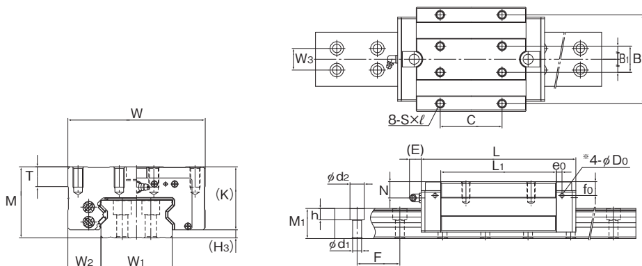
SRW70~100LR型
