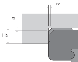
LM滑块的肩部
