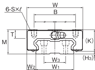
HRW27~50CR/CRM型
