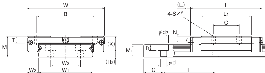
RSX15WM型
