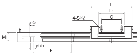
SRS15M/N、20M、25M型
