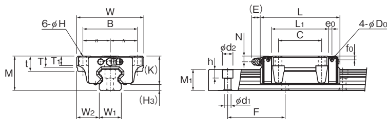
HSR20~35CB/HB/CBM/HBM型
