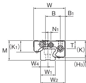
GSR15T/V型
