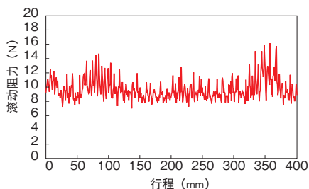
全钢球品 #25滚动阻力变动数据 (垂直使用、进给速度: 1mm/sec)
