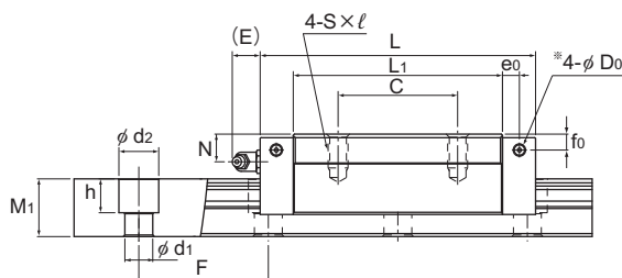
SVR-R型
