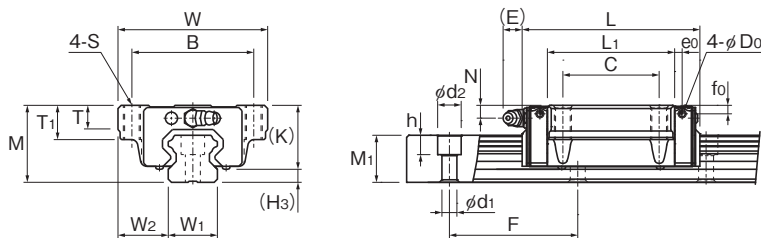
HSR15~35A/LA/AM/LAM型
