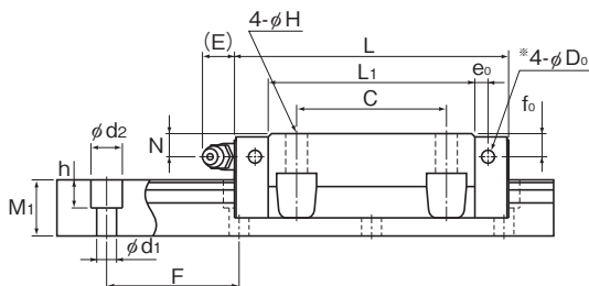
NR-B型、NRS-B型
