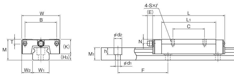
RSR15、20M1V/M1N型
