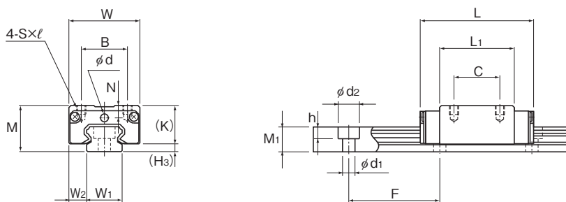
HSR8、10RM型
