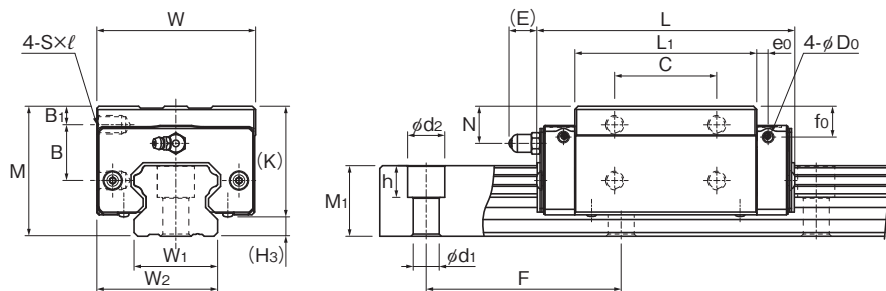
HSR45~65YR/XYR型
