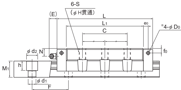
SVR-LC型
