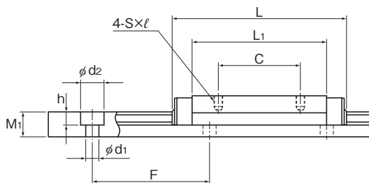
RSR9、12M1WV/M1WN型
