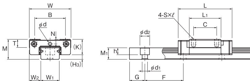
RSX7~12M型
