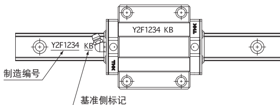
图12 基准侧的LM轨道(例: HSR-A型)
