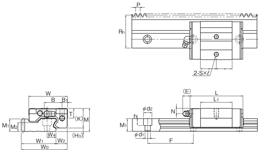
GSR25V-R型
