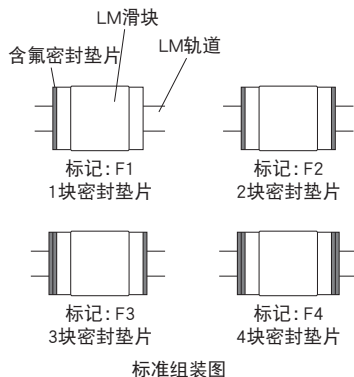
标准组装图
