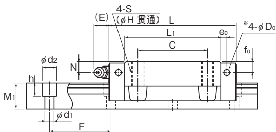
NR-CX型
