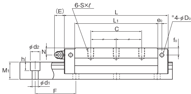
NRS-LRX型
