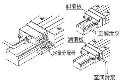
结构图
