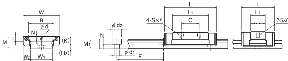
SRSTWM/WN、9WM/WN、12WM/WN型
