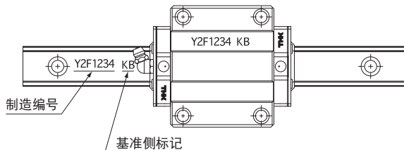
图16 基准侧的LM轨道(例: HSR-A型)
