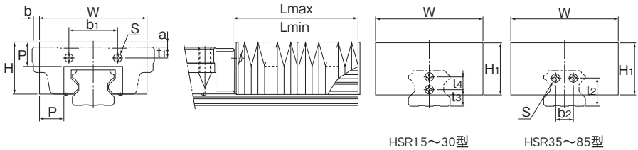
HSR15~30型 HSR35~85型
