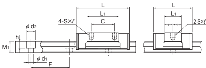
SRS7M/N、9XM/XN、12M/N型
