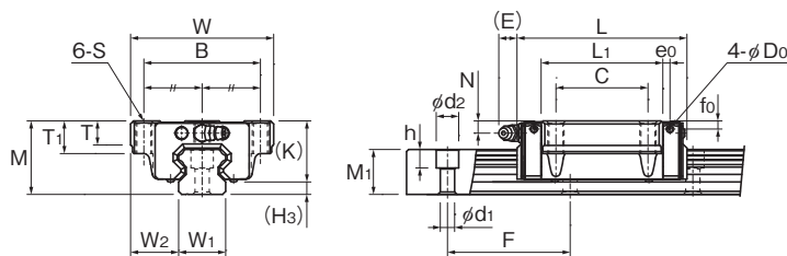
HSR20~35CA/HA/CAM/HAM型
