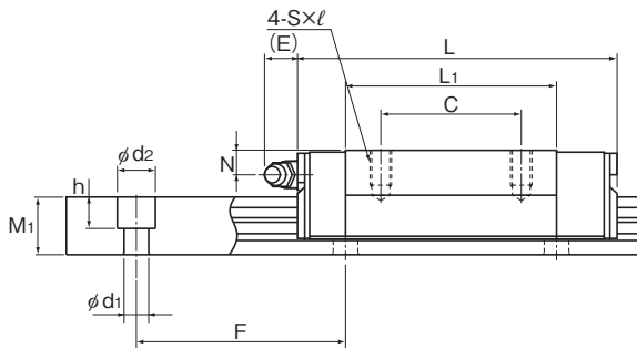
GSR15~35T型
