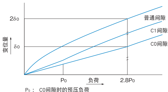
图10 刚性数据
