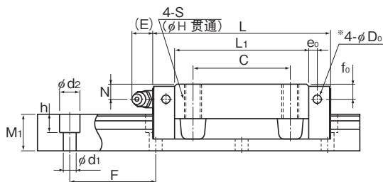
NRS-CX型
