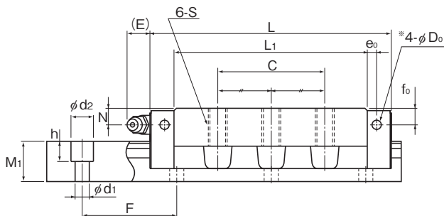
NR-LA型、NRS-LA型
