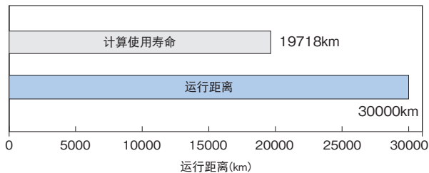
SHS65LVSS 高速耐久试验数据
