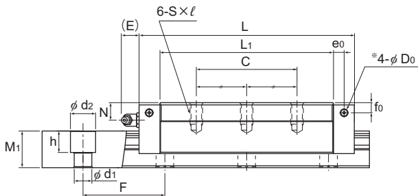
SVS-LR型
