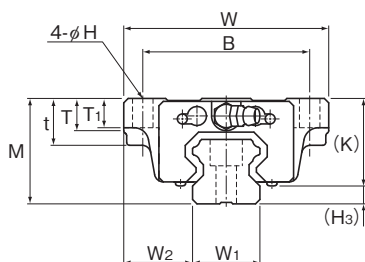
HSR15、25~35M1B/M1LB型
