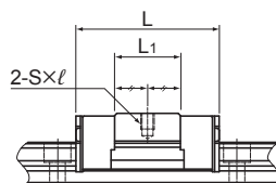
SRS15S型
