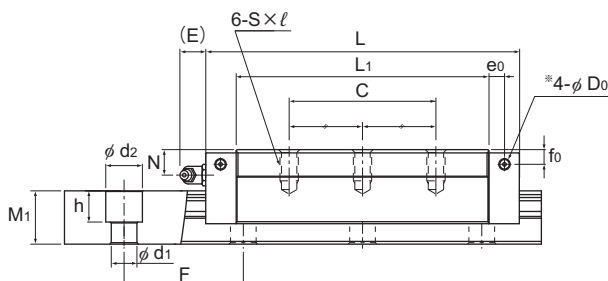
SVR-LR型
