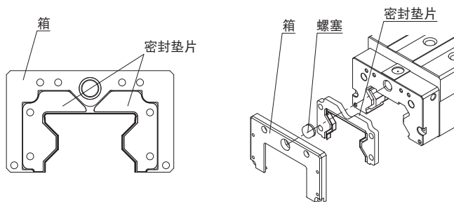
部件构成
