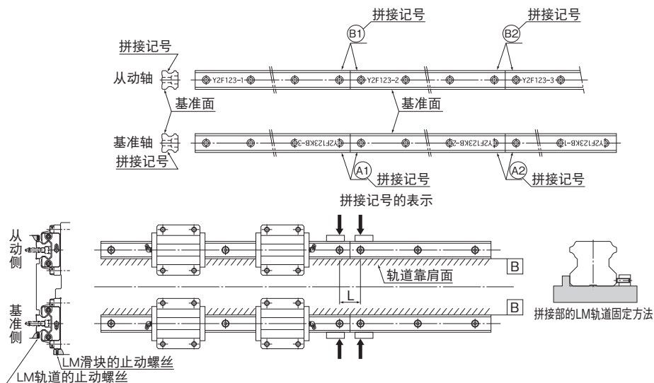
图23 拼接使用
