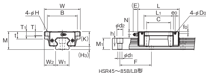
HSR45~85B/LB型
