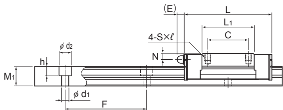
SRS15GM/GN、20GM、25GM型
